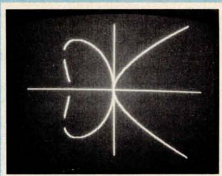
Y = \sqrt{(-2x^2 - 3x)/4 + \sqrt{(x^3 - x^4 + ((2x^2 + 3x)^2)/4)}}
